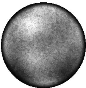
Pluto
