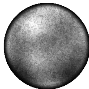
Pluto
