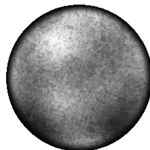
Pluto
