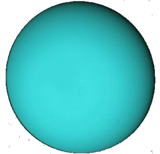
Uranus
