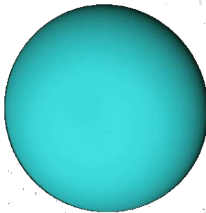
Uranus
