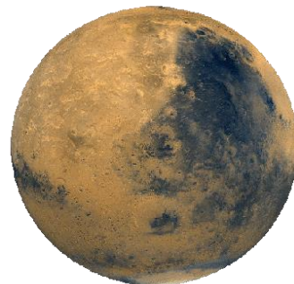
Mars
