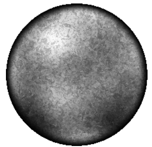
Pluto
