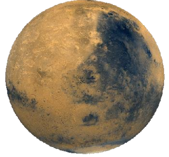
Mars
