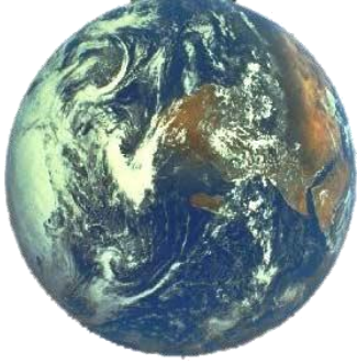
Earth
