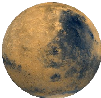
Mars
