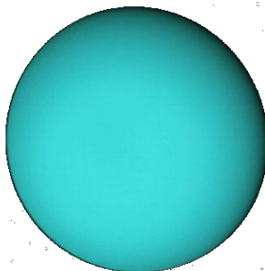
Uranus
